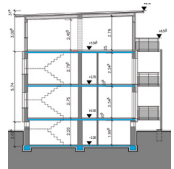
Schnitt A-A Neu
